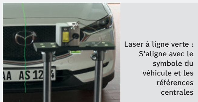
Réglage de la hauteur au laser selon le plancher
